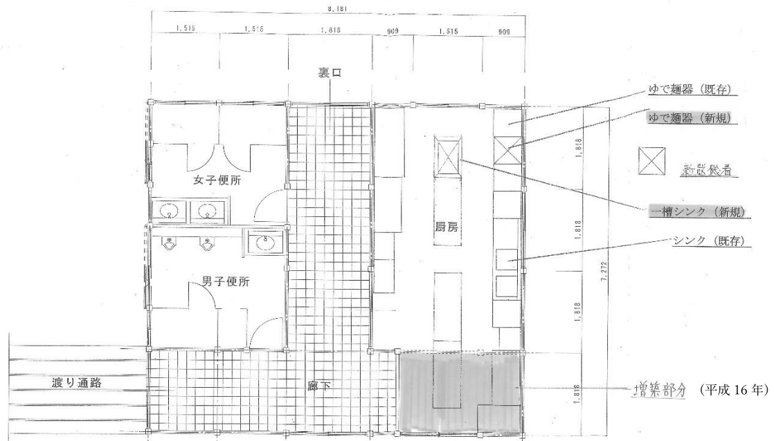
旧佐々木家住宅 図面（厨房、トイレ、渡り廊下）
