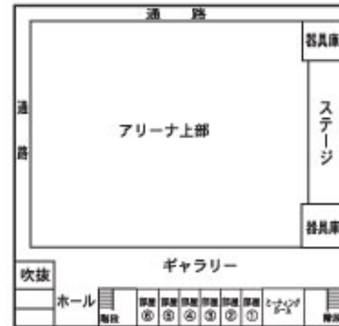
2階平面図
