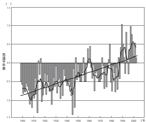
日本における年平均気温の経年変化(1898~2002年)
